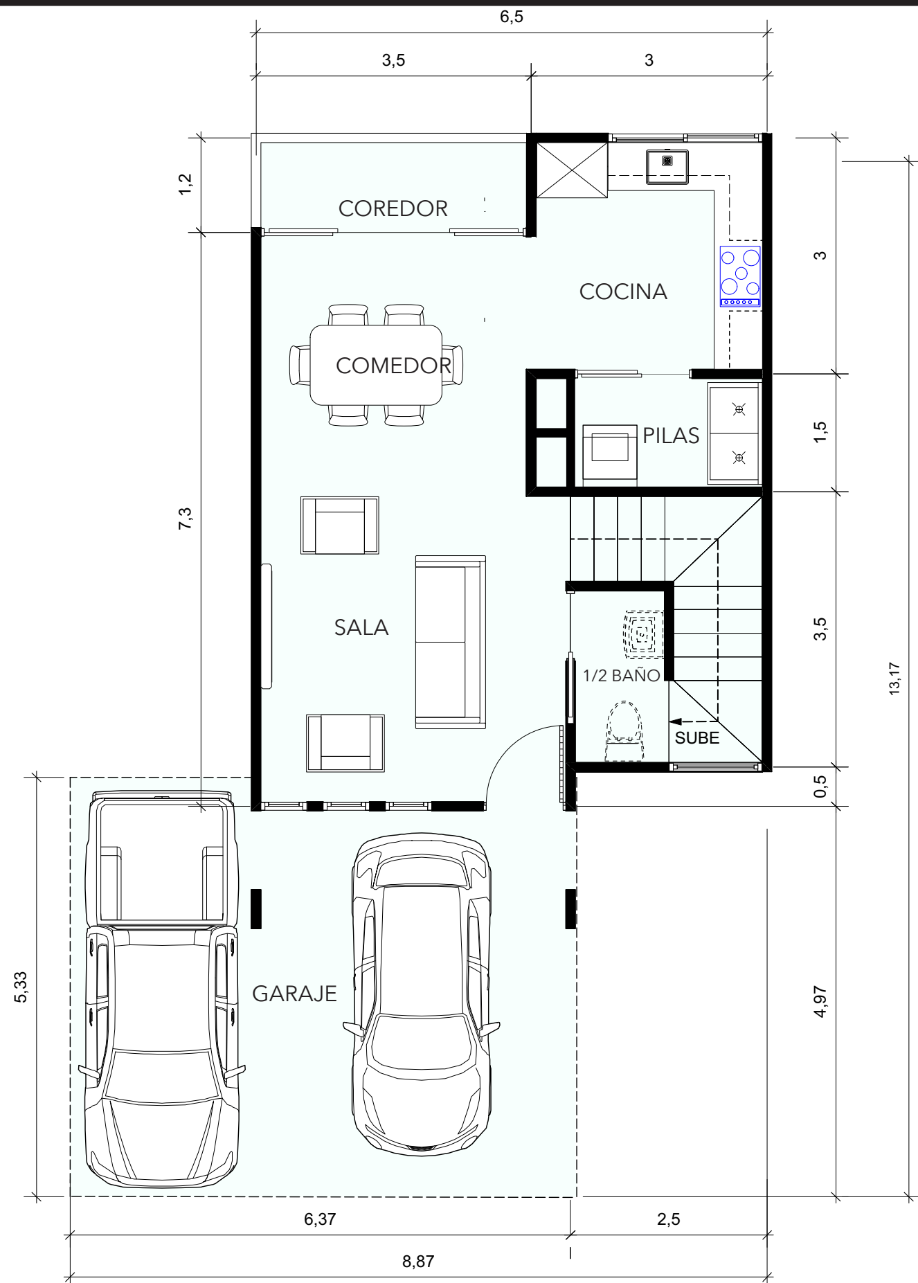
PLANTA ARQUITECTONICA PRIMER NIVEL
