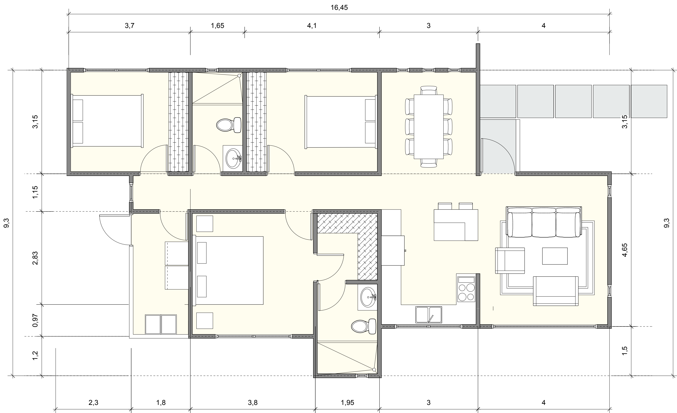
PLANTA ARQUITECTONICA CON 3 DORMITORIOS
