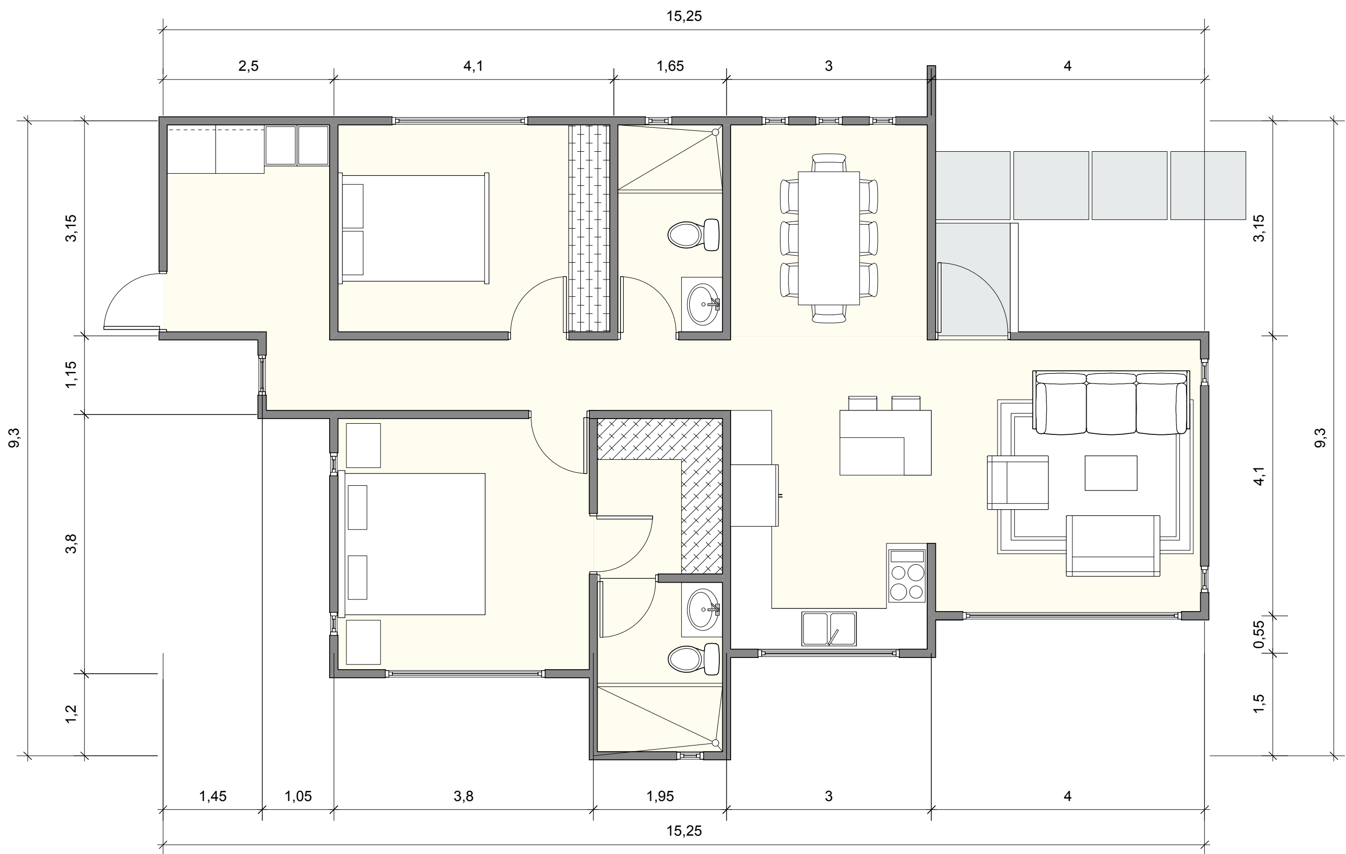
PLANTA ARQUITECTONICA CON 2 DORMITORIOS
