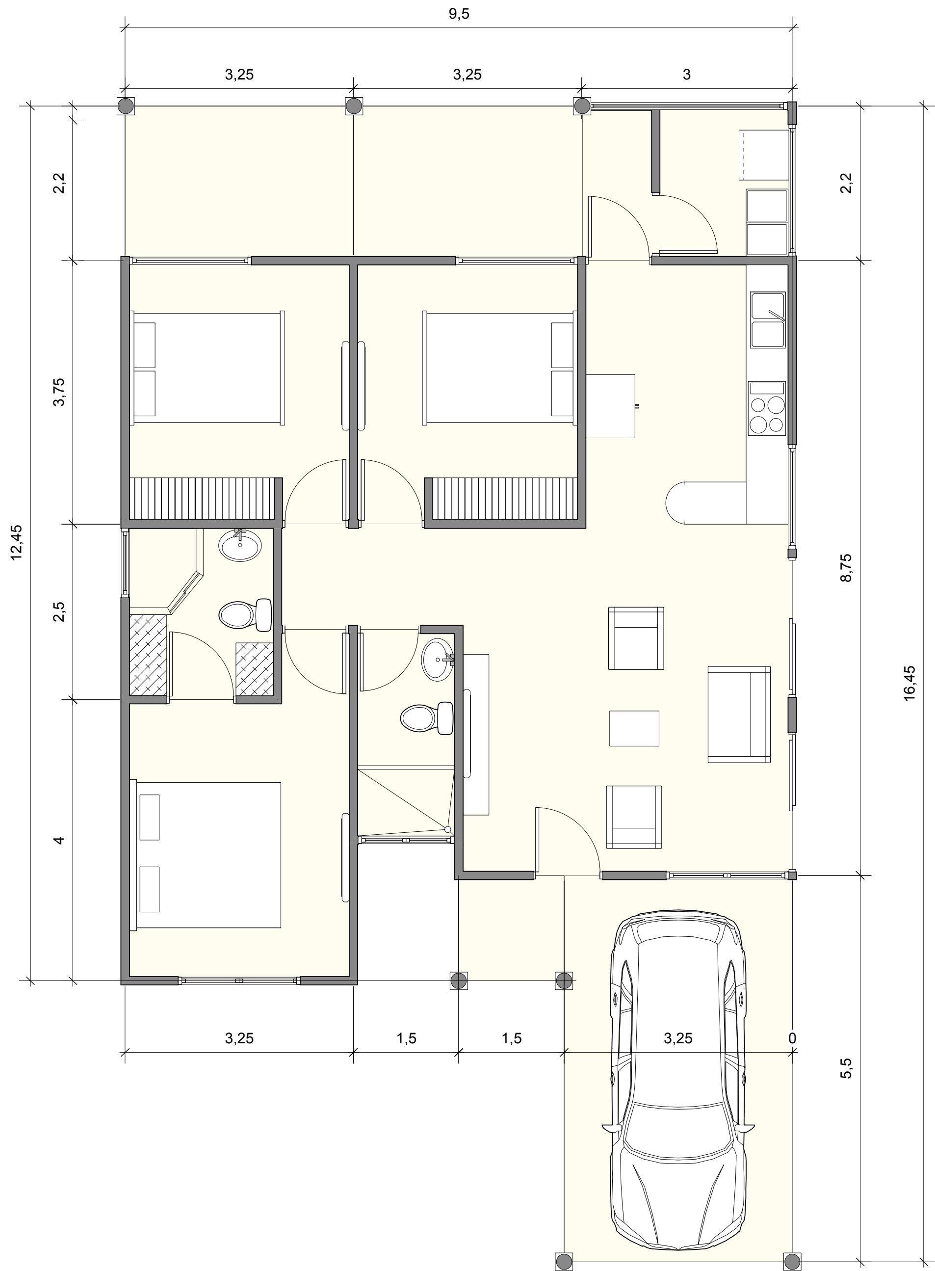
PLANTA ARQUITECTONICA
