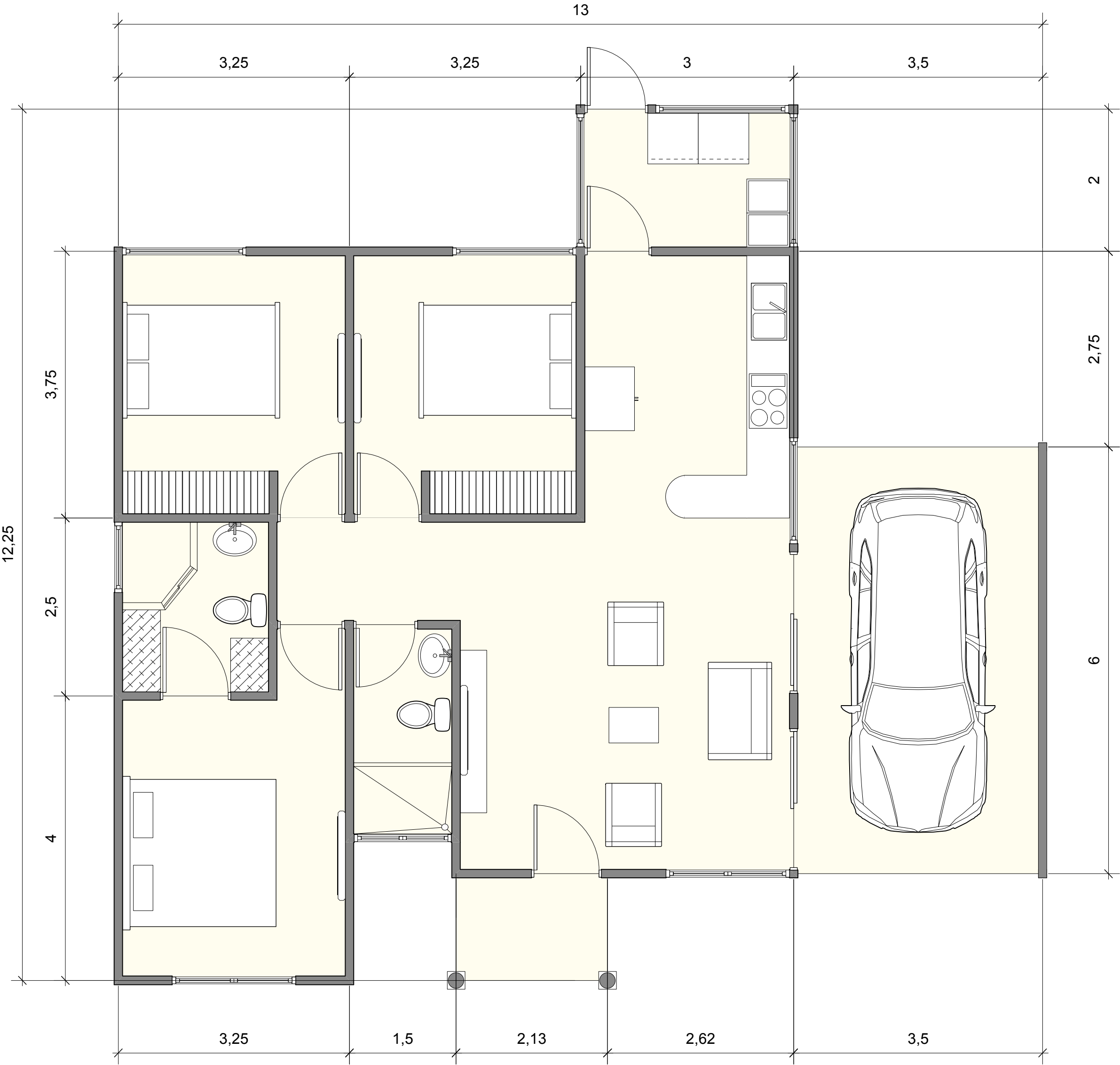
PLANTA ARQUITECTONICA
