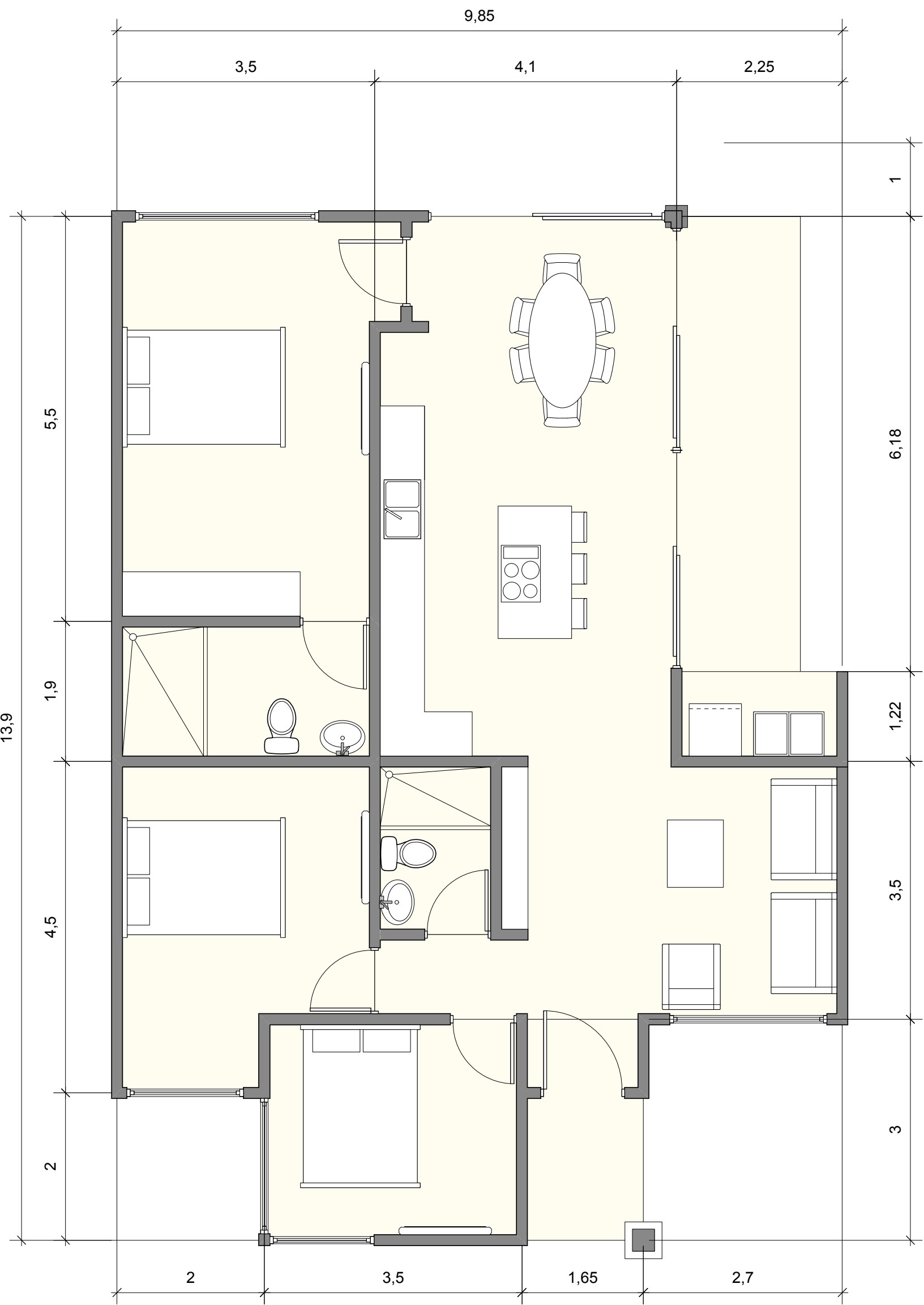
PLANTA ARQUITECTONICA
