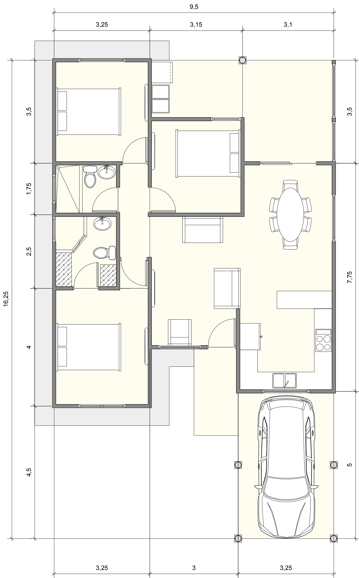
PLANTA ARQUITECTONICA
