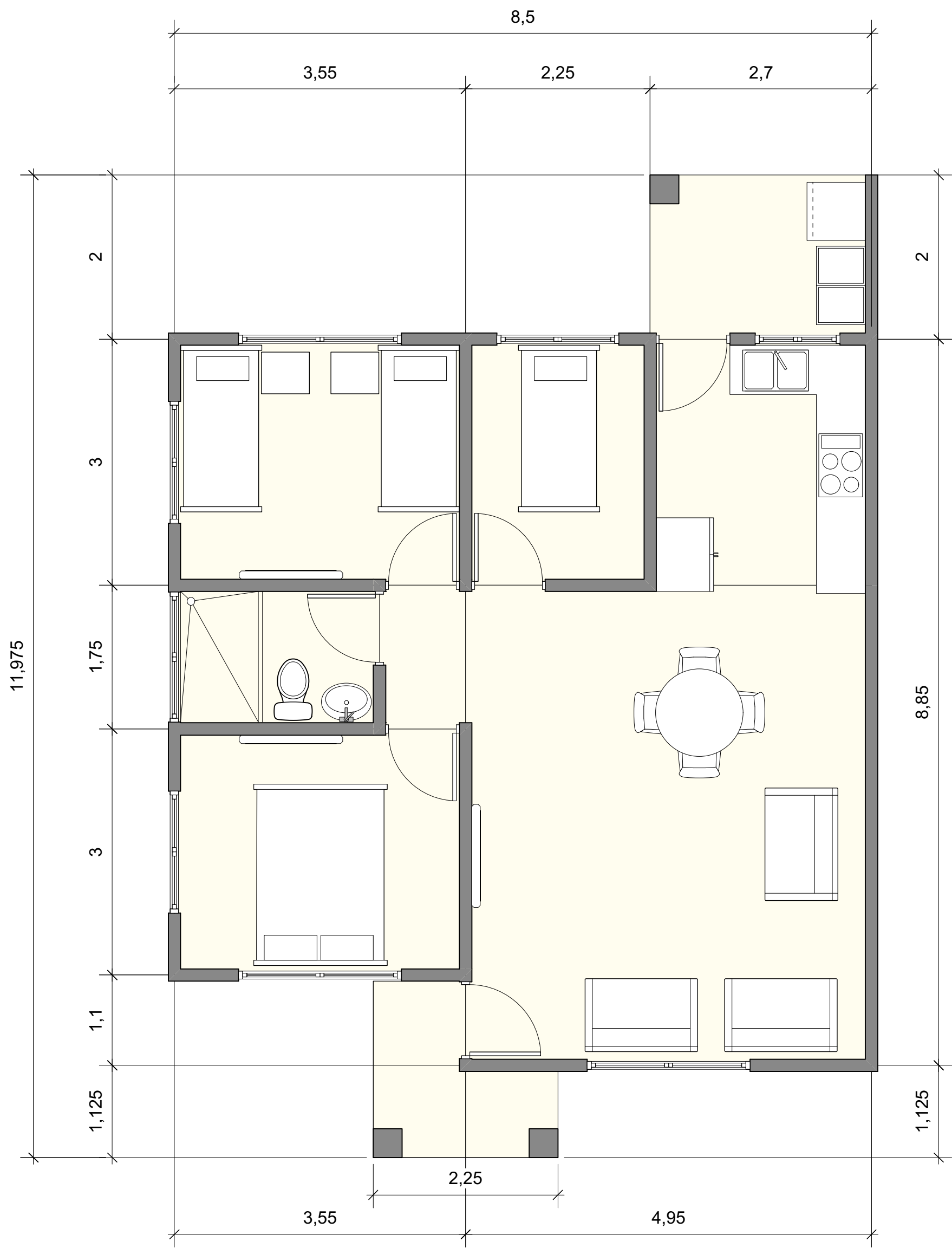
PLANTA ARQUITECTONICA
