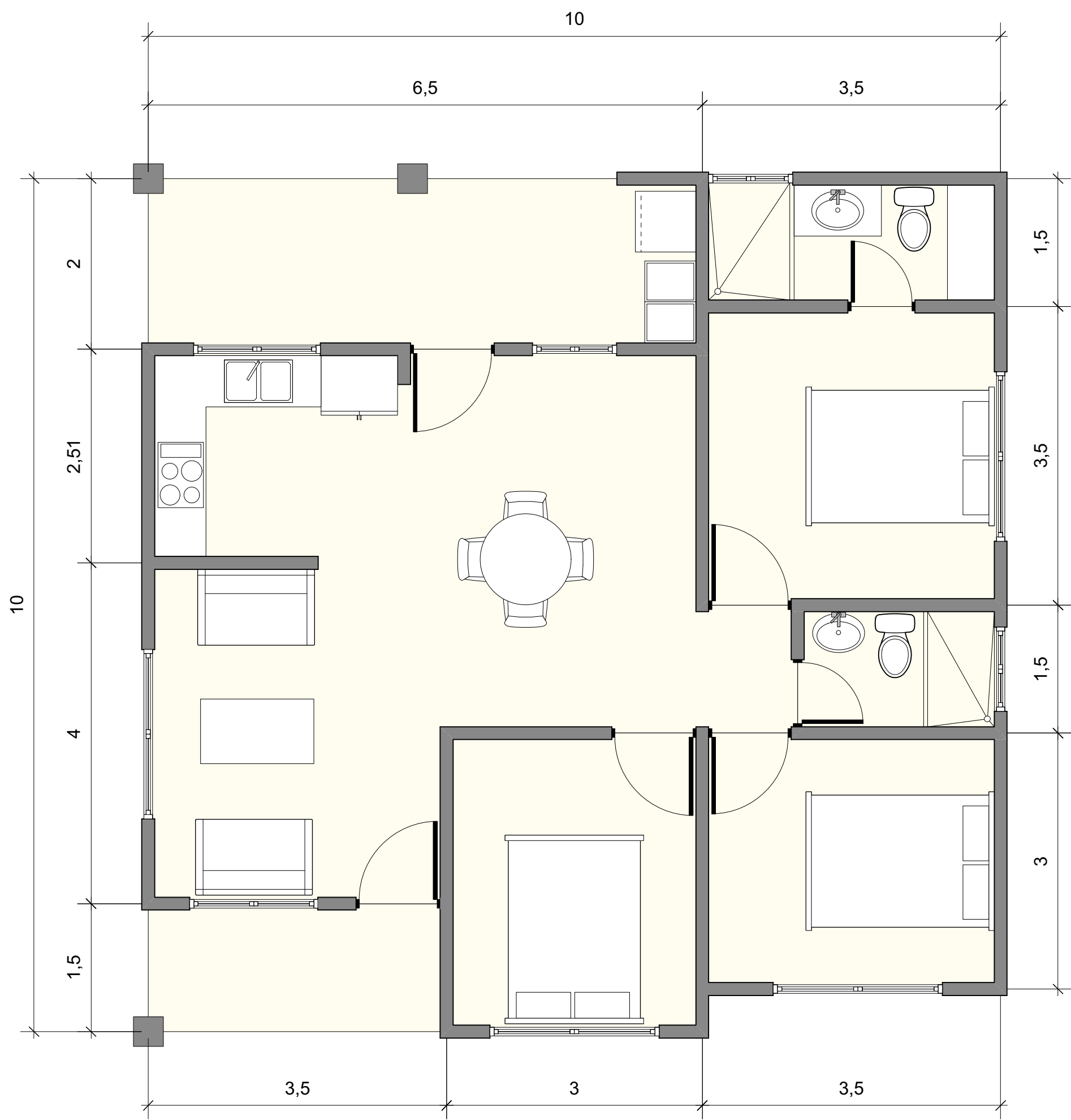
PLANTA ARQUITECTONICA
