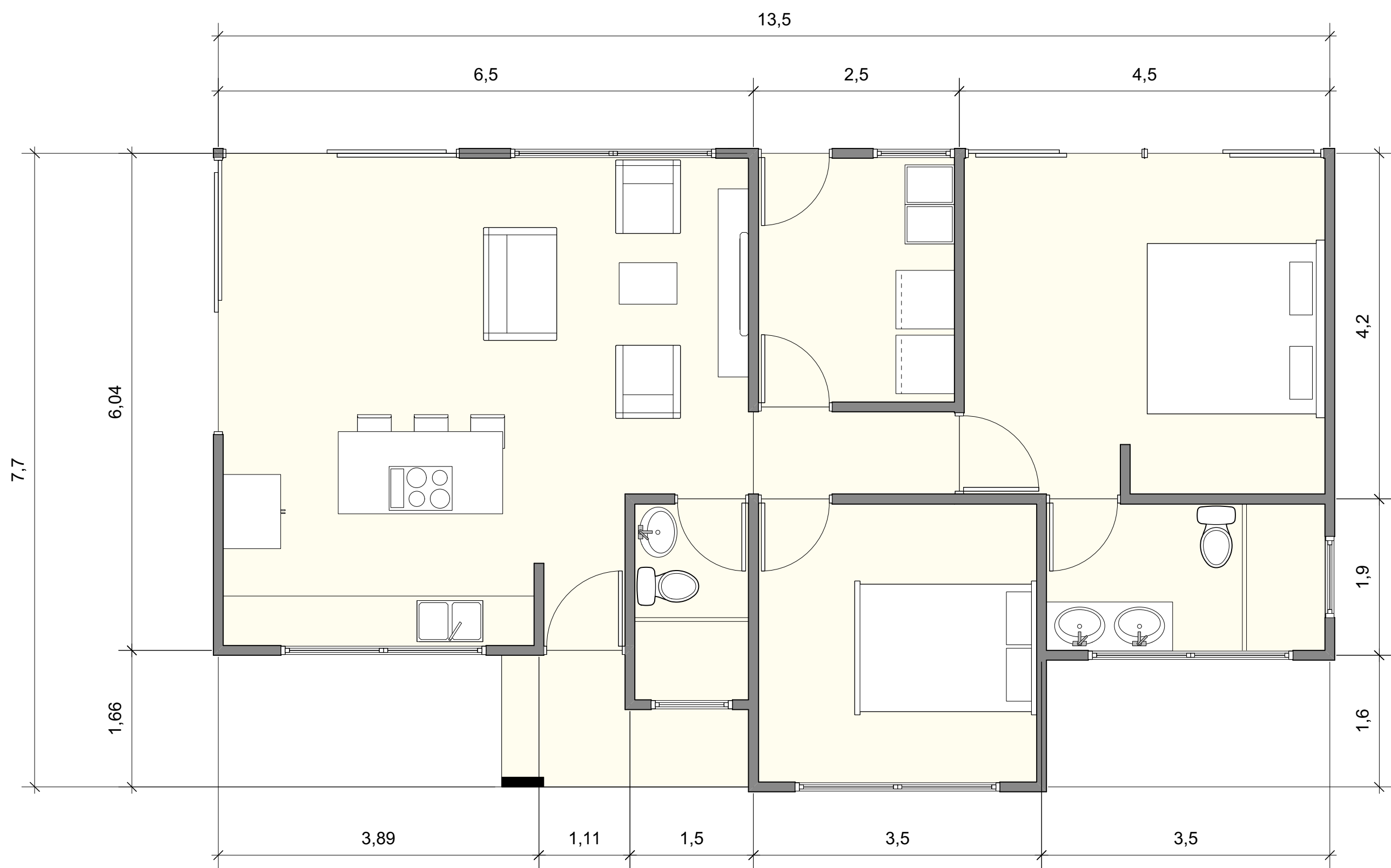
PLANTA ARQUITECTONICA VERSION ECONOMICA EN 2 DORMITORIOS
